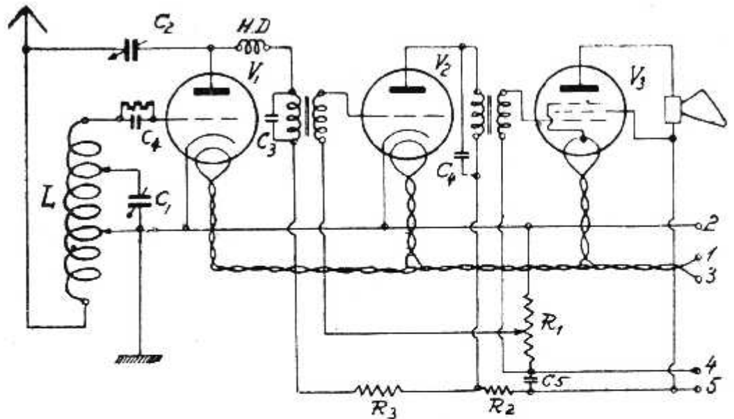
Principe schema van den handigen driepitter
