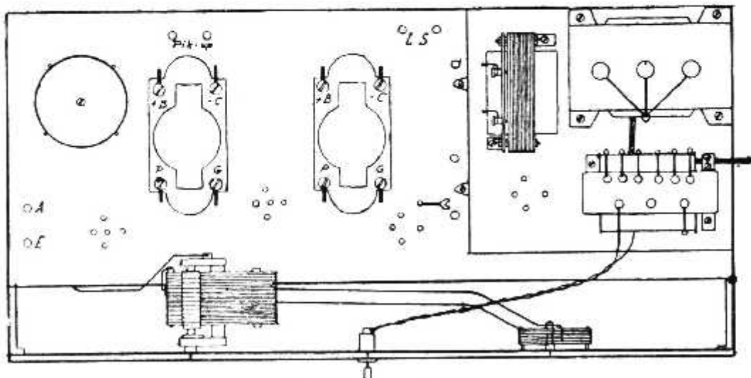
Opstelling der onderdeelen
