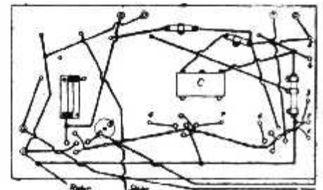
Schets der verbindingen onder de grondplank
