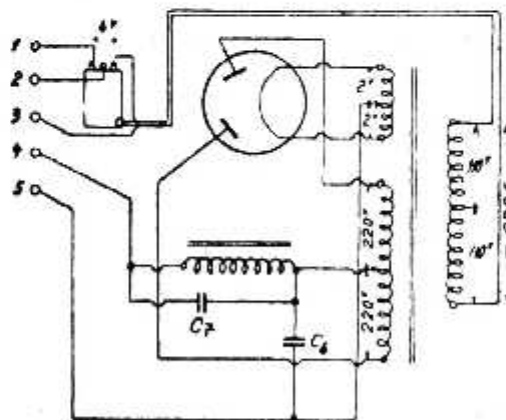
De schakeling van het „sterkstroom“ gedeelte
